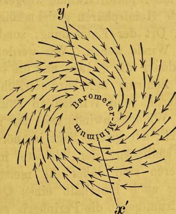
Fig. 28b. Antizyklonen und Zyklonen auf der südlichen Halbkugel.
