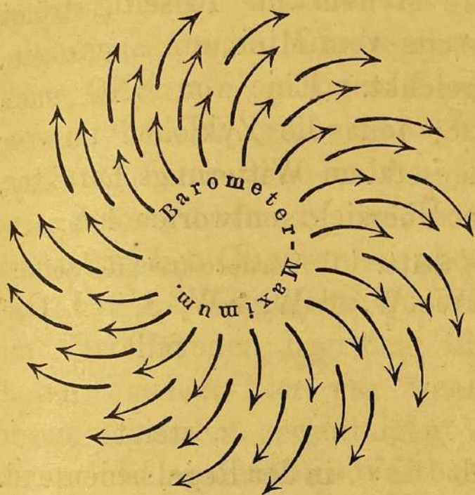
Fig. 28a. Antizyklonen und Zyklonen auf der nördlichen Halbkugel.
