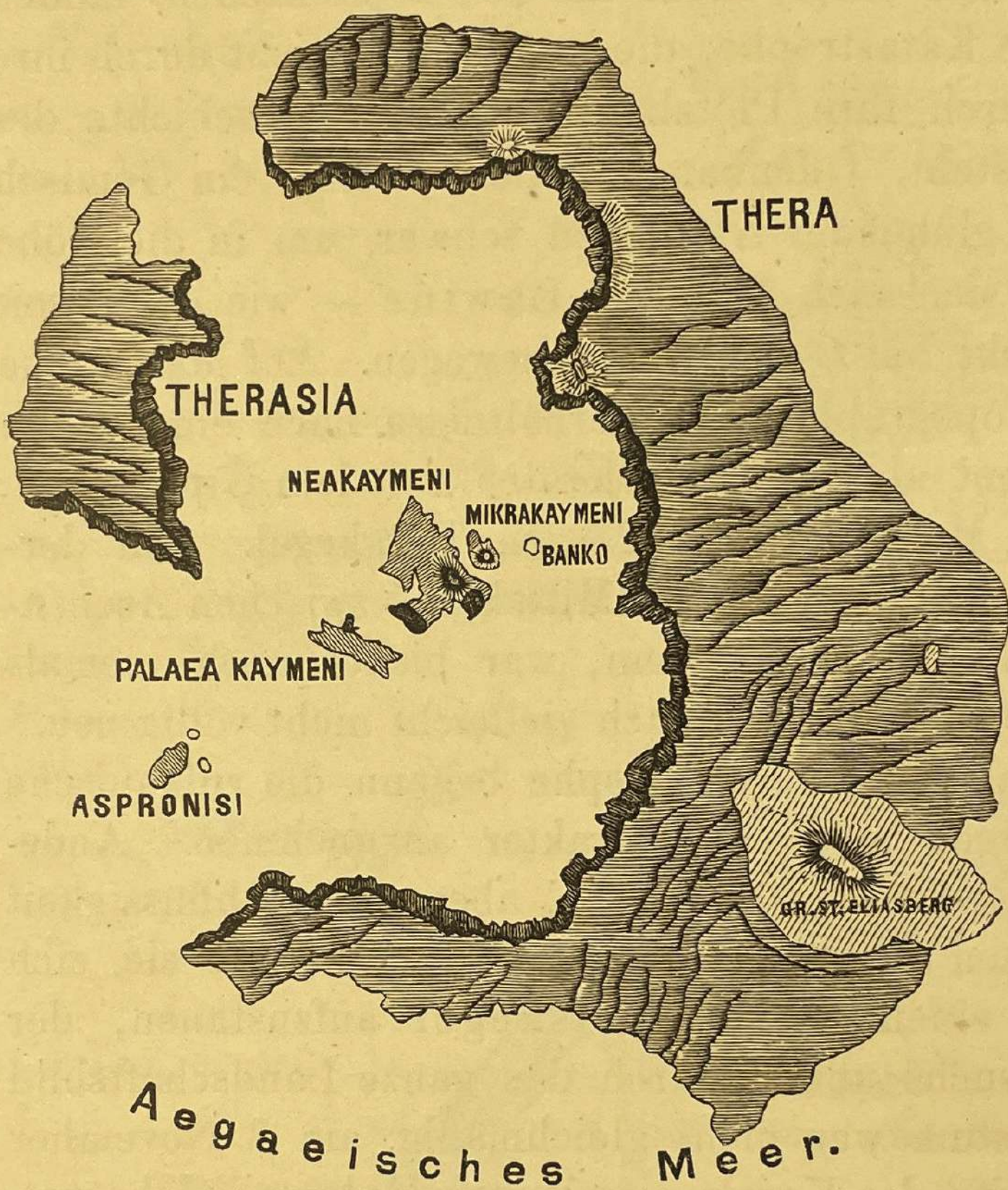
Fig. 100. Santorin im Jahre 1866 nach v. SEEBACH.
