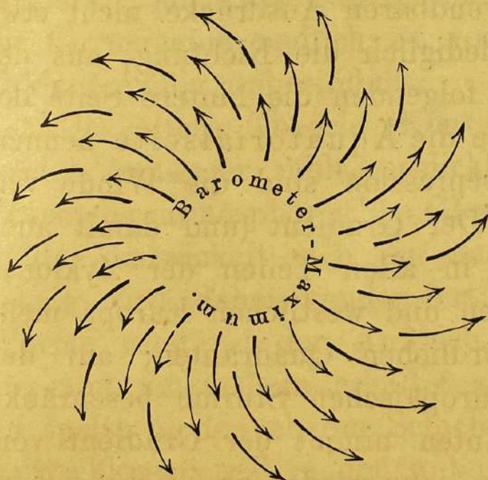
Fig. 28b. Antizyklonen und Zyklonen auf der südlichen Halbkugel.
