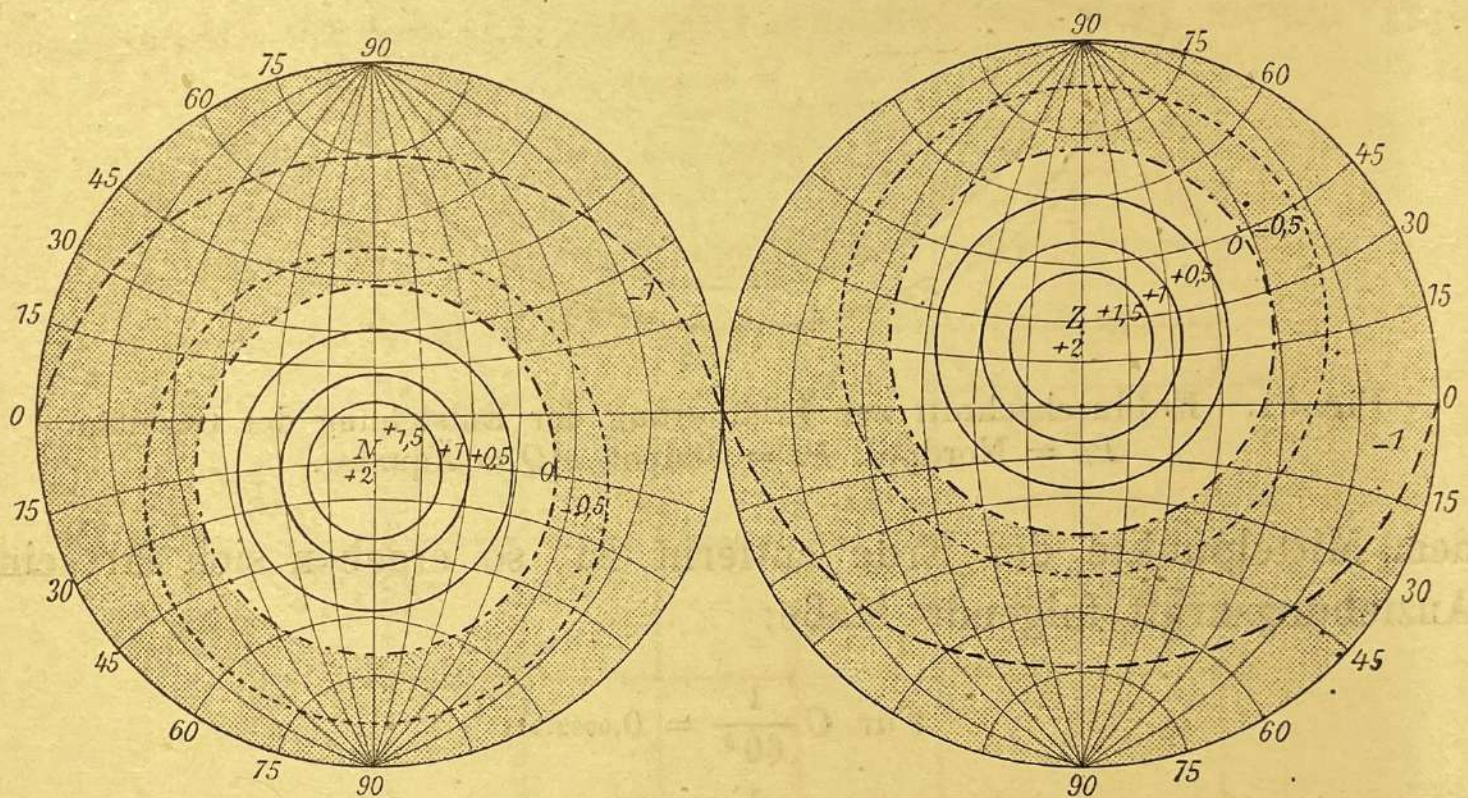
Fig. 62. Karte der Gleichgewichtszeiten nach G. H. DARWIN. 1
