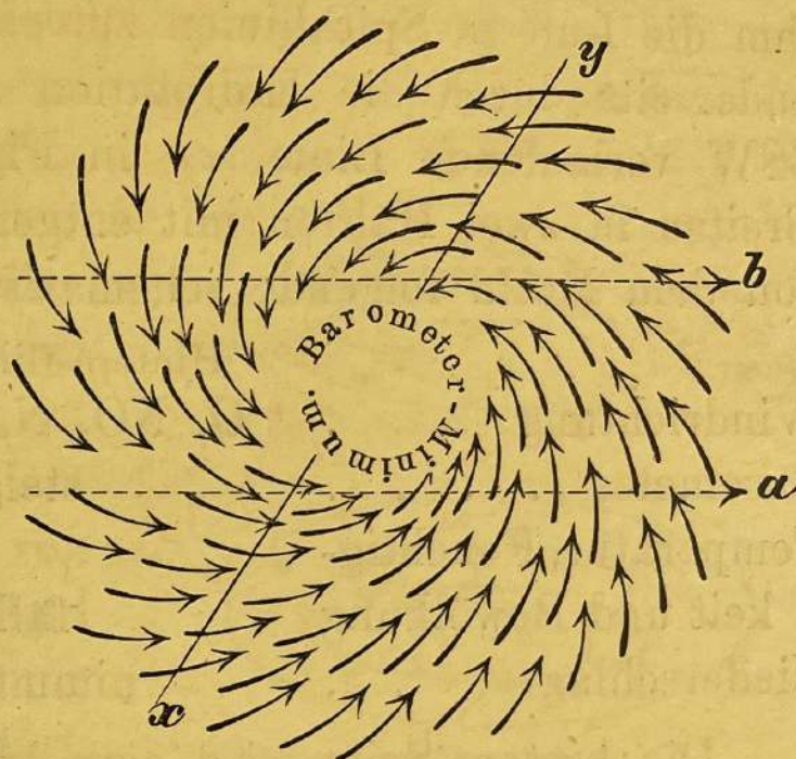
Fig. 28a. Antizyklonen und Zyklonen auf der nördlichen Halbkugel.
