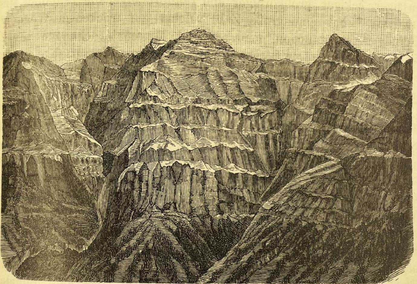
Fig. 116. Verwitterungsterrassen im Glärnisch-Gebirge nach BALTZER.
