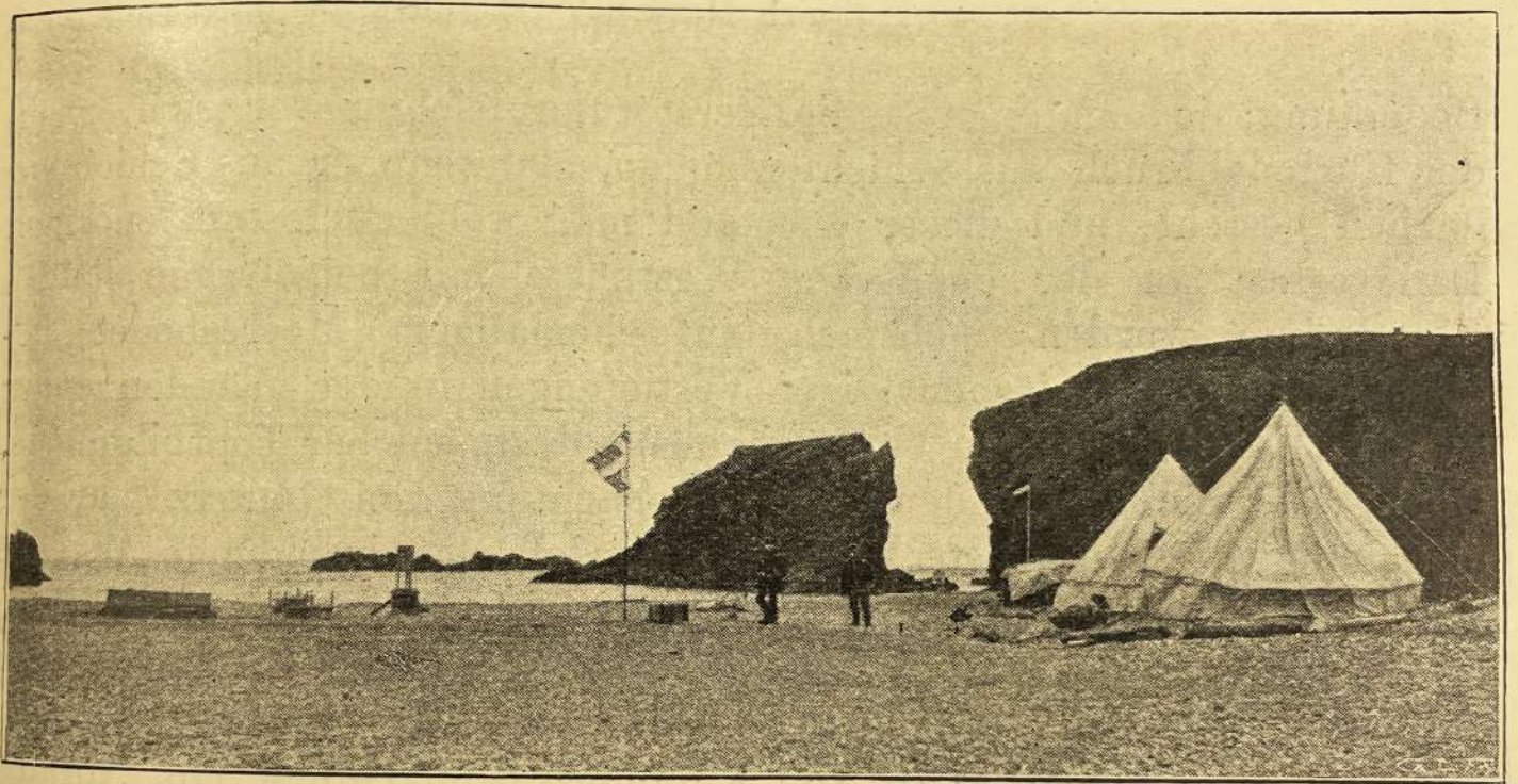
Fig. 169. Das Bürgermeistertertor auf der Bäreninsel 1899 nach G. ANDERSSON.
