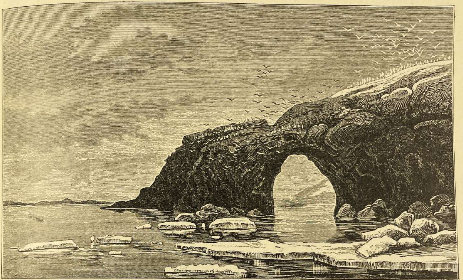
Fig. 168. Das Bürgermeisterter auf der Bäreninsel 1864 nach G. ANDERSSON.
